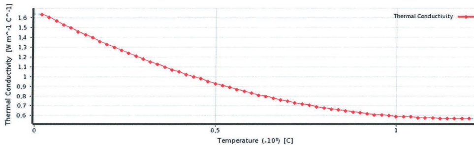
Diagramm 4: Beton Wärmleitfähigkeit
